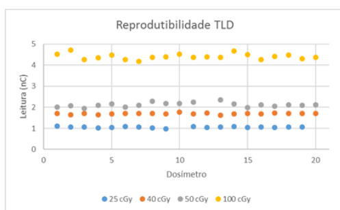
Figura 1: Leituras TLD para quatro grupos de dosímetros após a irradiação com diferentes doses (25, 40, 50 e 100 cGy).
